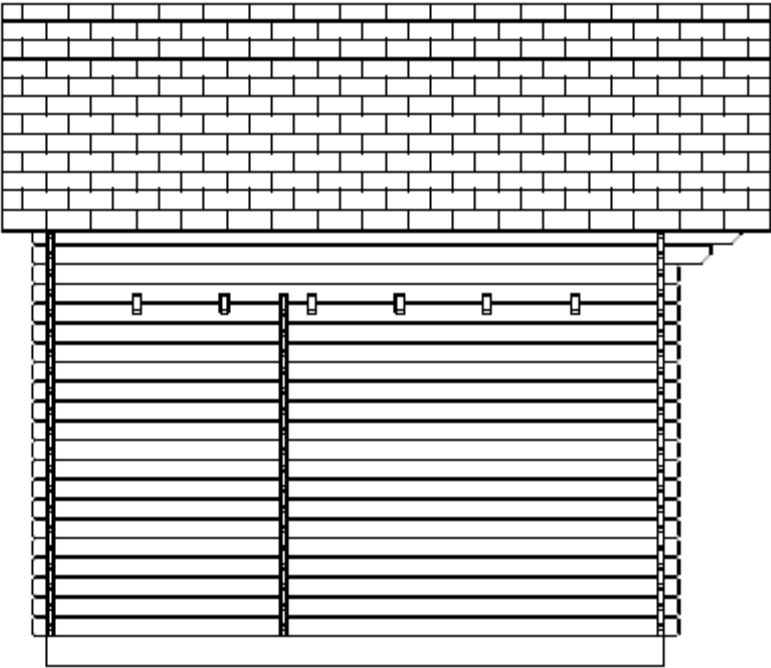
COTE GAUCHE
