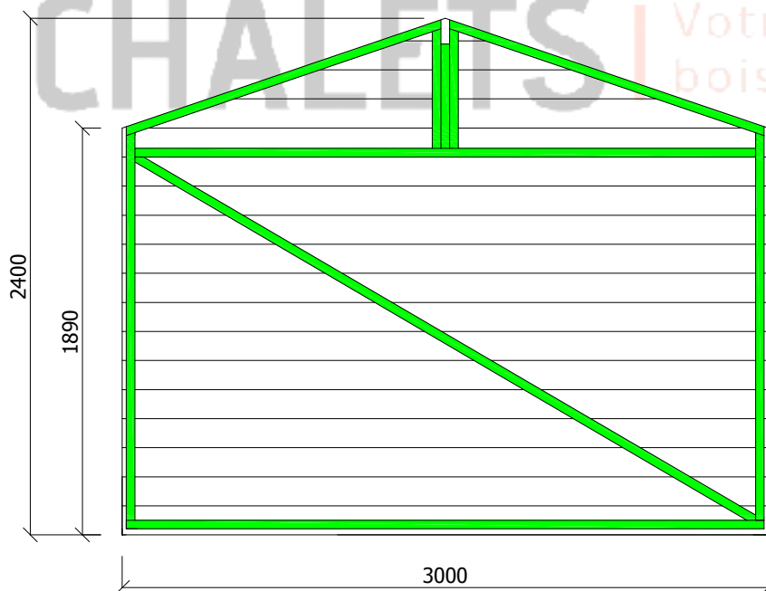
MURS A ET B
